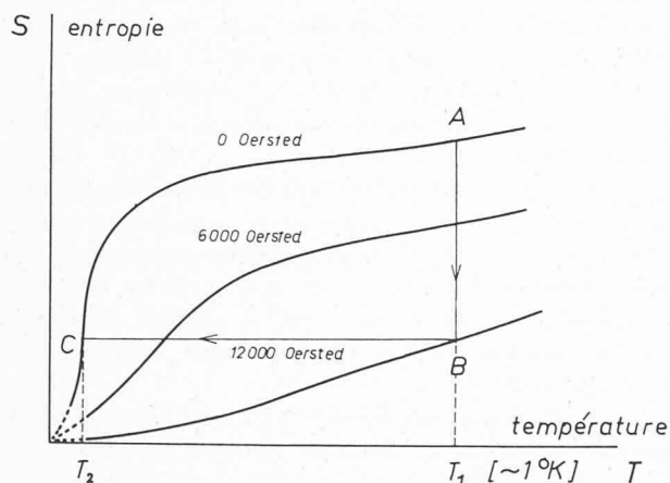
Fig. 2. — Diagramme entropie-température d'un sel paramagnétique pour différents champs magnétiques extérieurs. Le chemin suivi lors de la désaimantation adiabatique est marqué par les points ABC.
