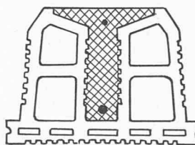
Coupe de la poutrelle préfabriquée : béton pervibré, coffré par la terre cuite, nervure en T rationnelle; isolation parfaite.
