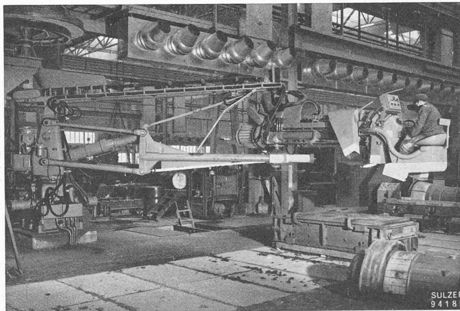
Fig. 9. — Sandlinger stationnaire dans le moulage des pièces moyennes.
