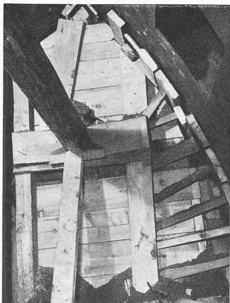
Fig. V/7. — Etayage du front d'attaque, sous le faite.
