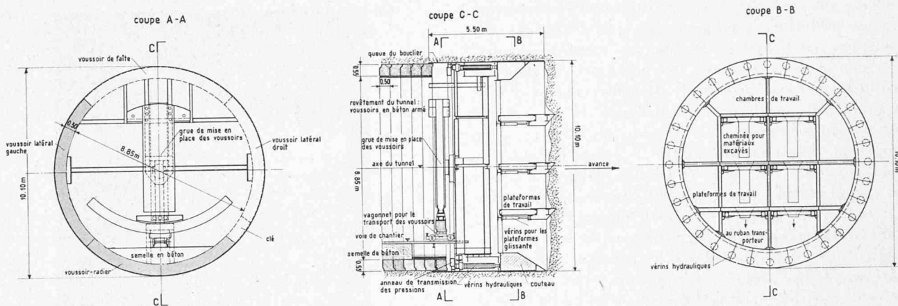
Fig. V/5. — Coupe en long et en travers du bouclier.
