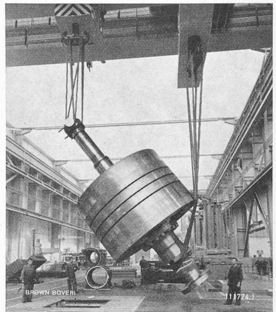
Fig. 5. — Manutention d'une roue polaire d'un alternateur destiné à la centrale de Tokke (Norvège), à l'aide de deux ponts roulants de 60 t et un de 150 t.
