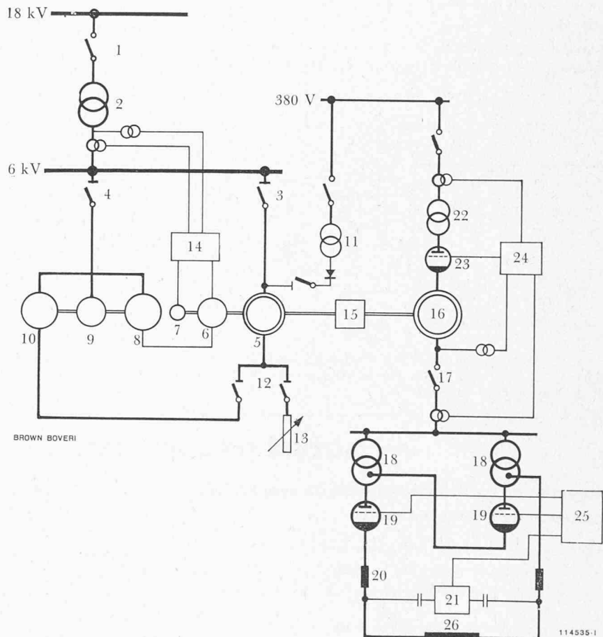
Fig. 1. — Schéma unipolaire de l'installation d'alimentation de l'électro-aimant.
