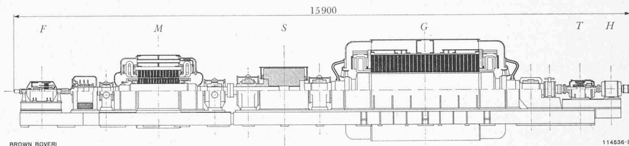
Fig. 2. — Vue en coupe du groupe convertisseur.
