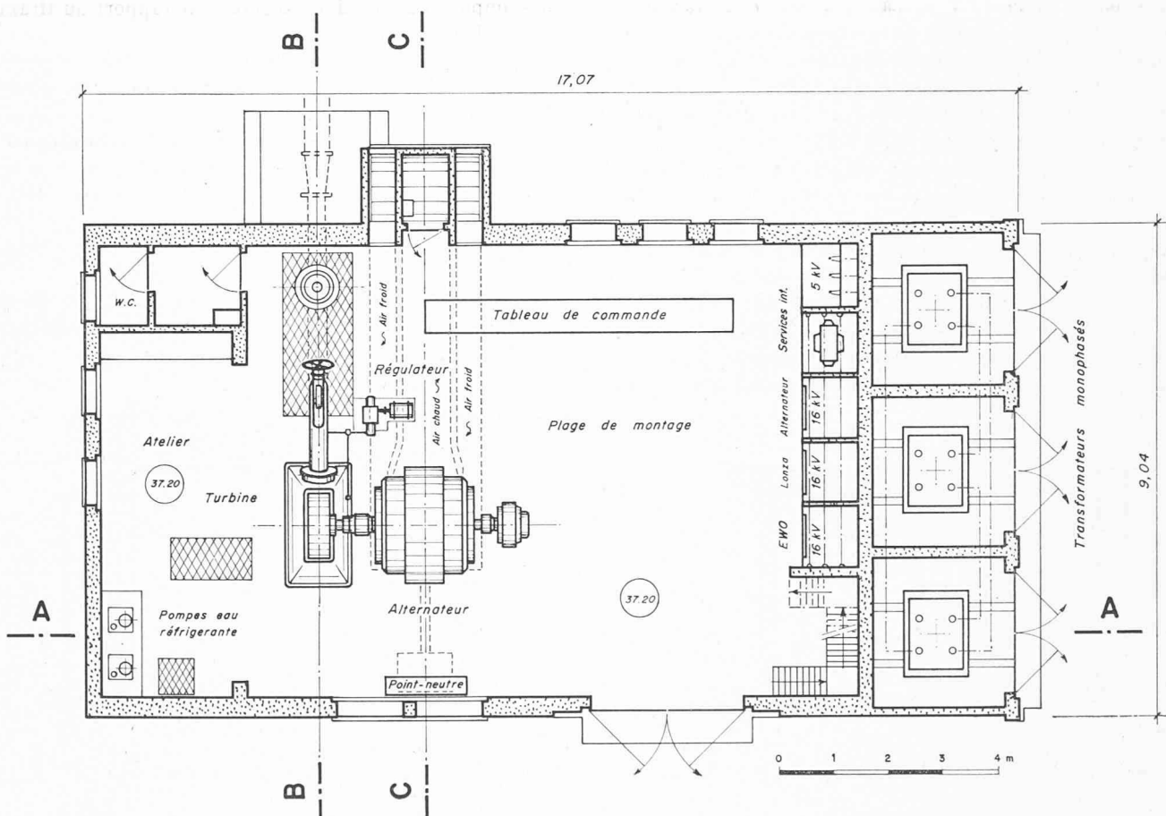
Fig. 11. — Centrale, plan.
