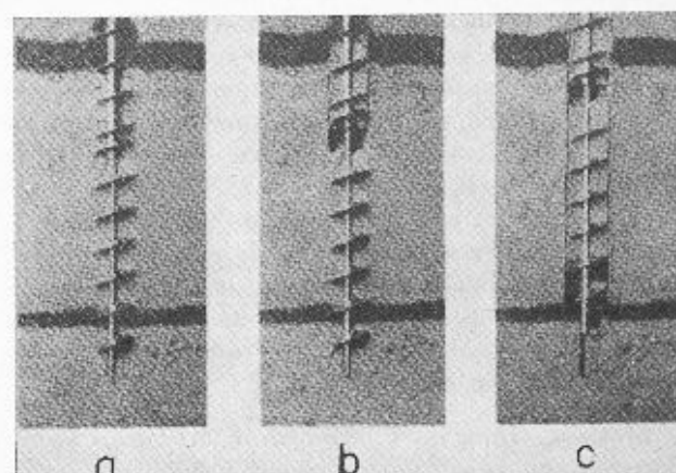
Fig. 7. — Tarière bipartite.
