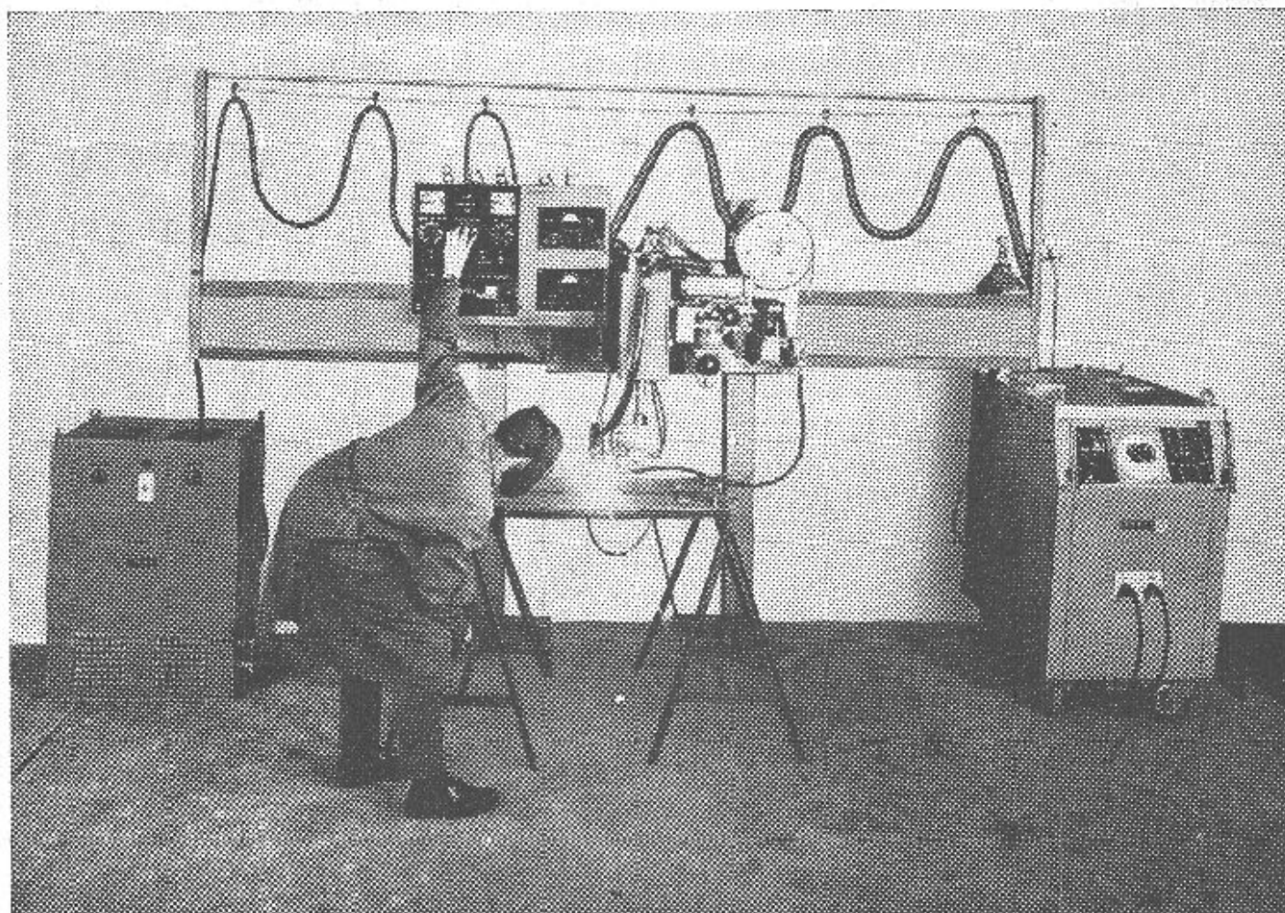
Installation de soudage automatique TIG, VOLTAFIX Sécheron.
