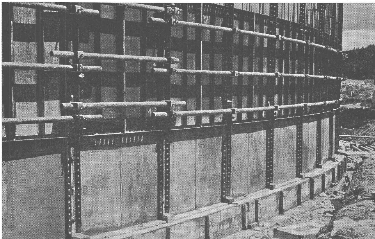
Coffrage grimpant
