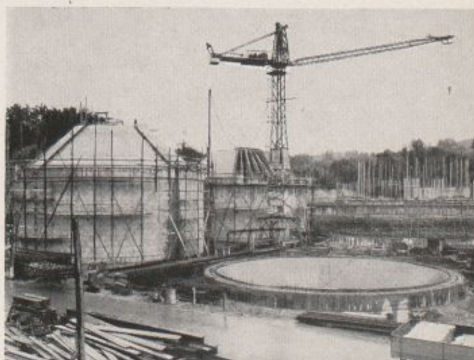
Fig. 13. — Station d'épuration des eaux du Werdhölzli à Zurich. Digesters
