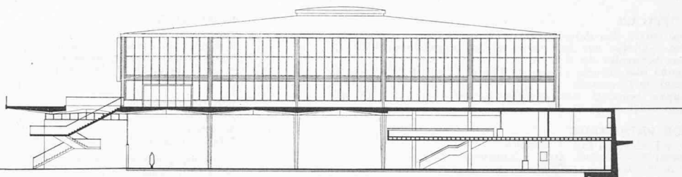
Coupe transversale entre pavillons.
