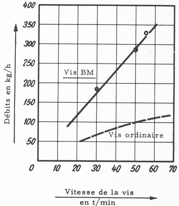
Fig. 4. — Extrudeuse BM 120, 18 D.
