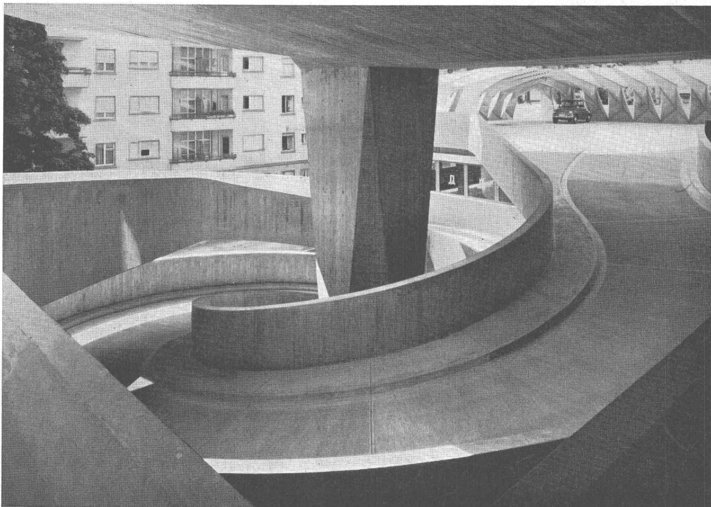
Rampe d'accès de la maison-tour « zur Palme » à Zurich. Chape en béton dur Korodur, exécutée par l'entreprise Heinr. Hatt-Haller S. A. à Zurich.
