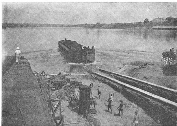
Fig. 4. — Lancement d'un chaland.
