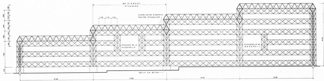
Fig. 9. — Coupe longitudinale de l'ossature du secteur C4.
