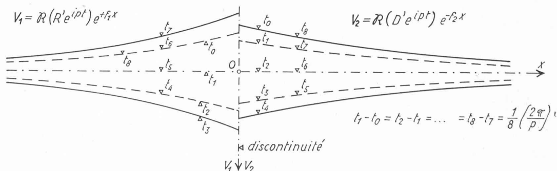
Fig. 3. — Onde stationnaire produite, au voisinage du point O où la section de la barre est discontinue, par une vibration incidente transversale.
