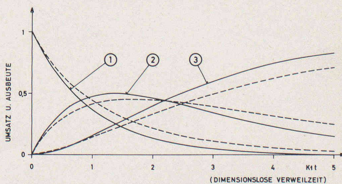
Fig. 1. — Débits et production d'une réaction en cascade de premier ordre dans un tube cylindrique.
