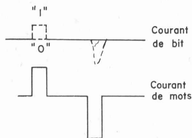
Fig. 13. — Lecture du mot dans le cas d'une mémoire à basculement total.
