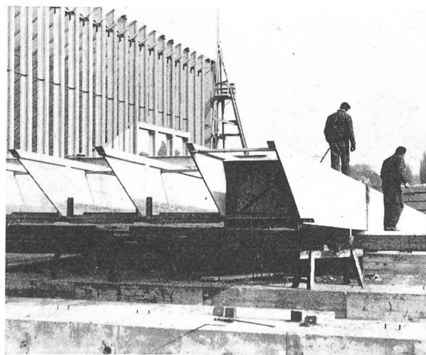
Fig. 13. — Diaphragme de raidissement d'une poutre caisson.
