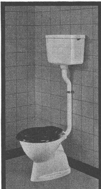
Réservoir de chasse GEBERIT-CPV no. 10.000 pour montage à mi-hauteur, avec tuyau de chasse no. 44.020 2" x 1 1/2", longueur 70 x 22 cm.
