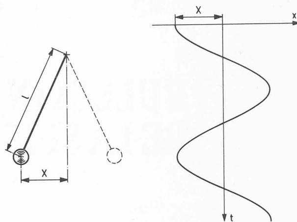
Fig. 2. — Oscillations d'un pendule.
