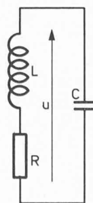
Fig. 3. Circuit oscillant avec pertes.
