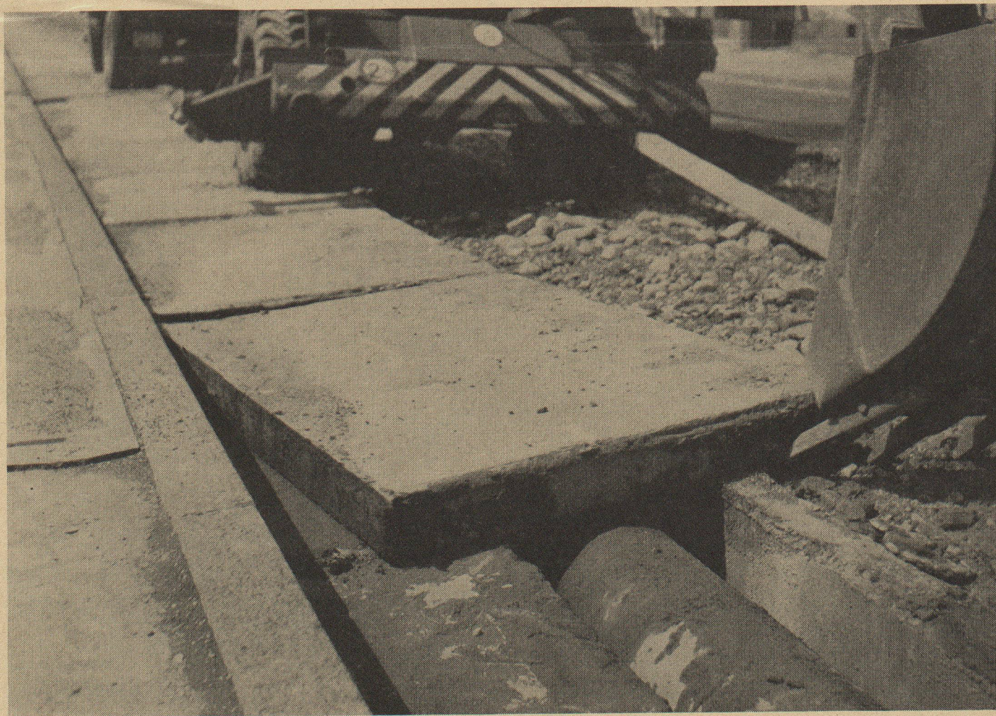
Réfection du tablier du pont de Pérolles à Fribourg au moyen du produit « Colma-fix ».
