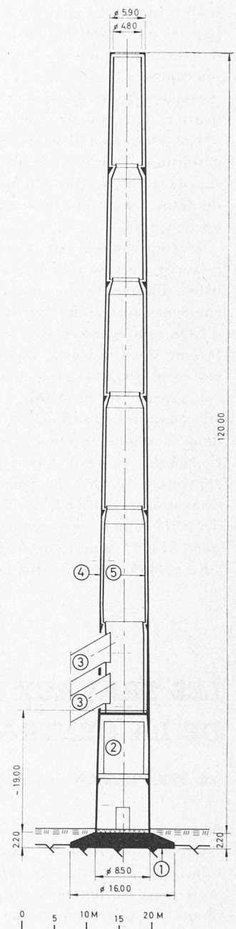
Fig. 1. Cheminée : coupe verticale. 1. Semelle de fondation — 2. Réservoir d'eau 220 m 3 . — 3. Carnaux. — 4. Manteau en béton armé. — 5. Revêtement intérieur de briques.
