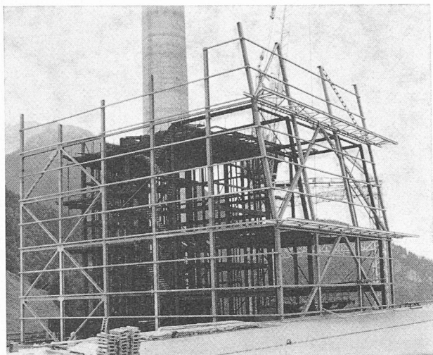
Fig. 6. — Montage du capot (structure en clair) autour de la chaudière terminée (structure sombre).
