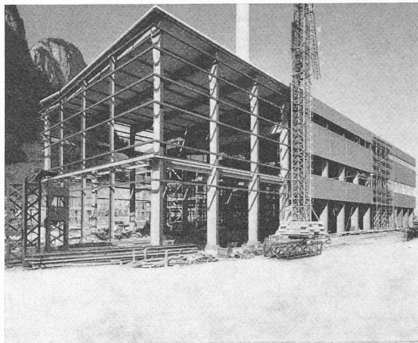
Fig. 8. — Extérieur de la salle des machines.
