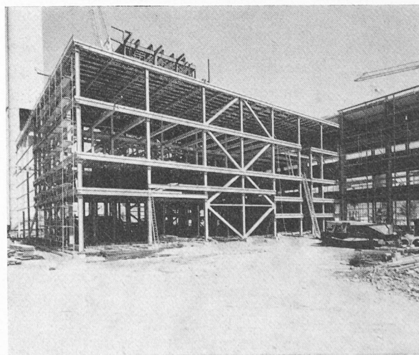
Fig. 9. — Bâtiment de commande vu depuis l'extérieur.
