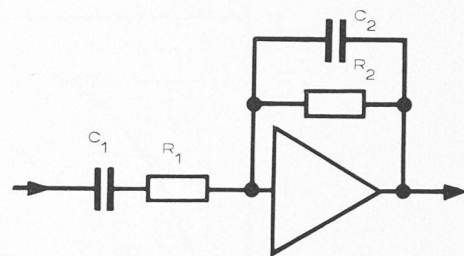
Fig. 4. — Périodemètre.
