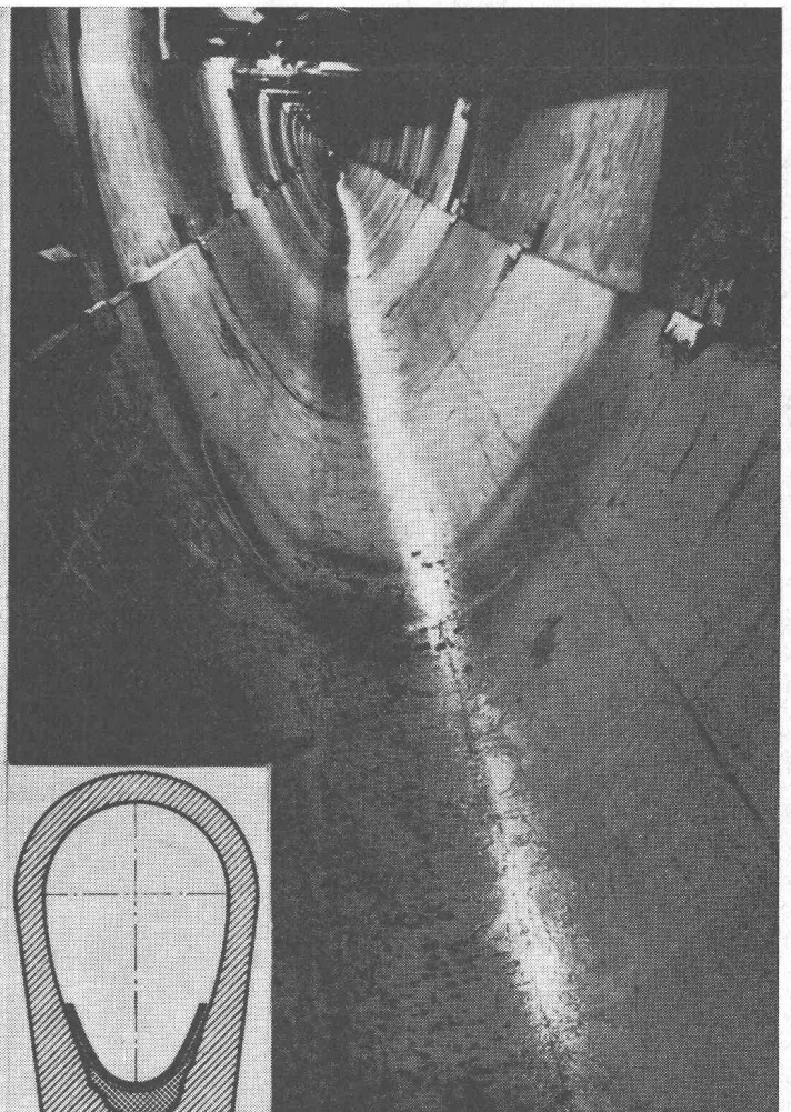
Réparation d'un égout au moyen d'éléments préfabriqués au mortier au liant synthétique (MZ)
