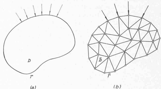
Fig. 10. — Disque sollicité par des forces coplanaires.
