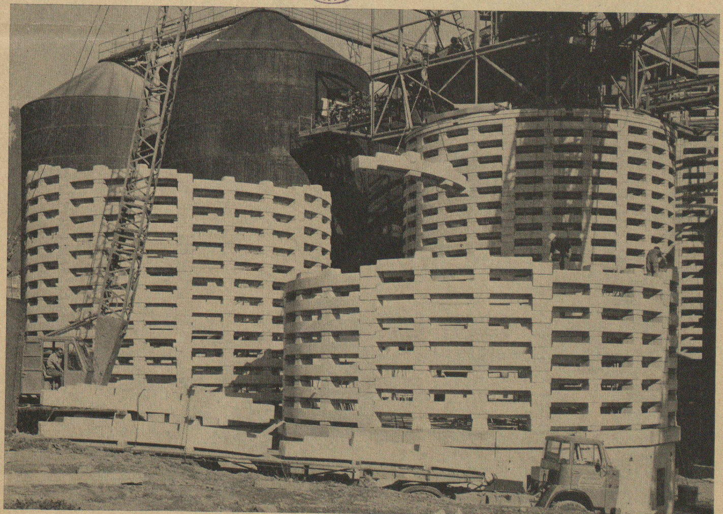
Silos en éléments de béton armé préfabriqués Fabrication et montage : Igéco S.A., Etoy Photo : Stamm & Saxod, Lausanne
