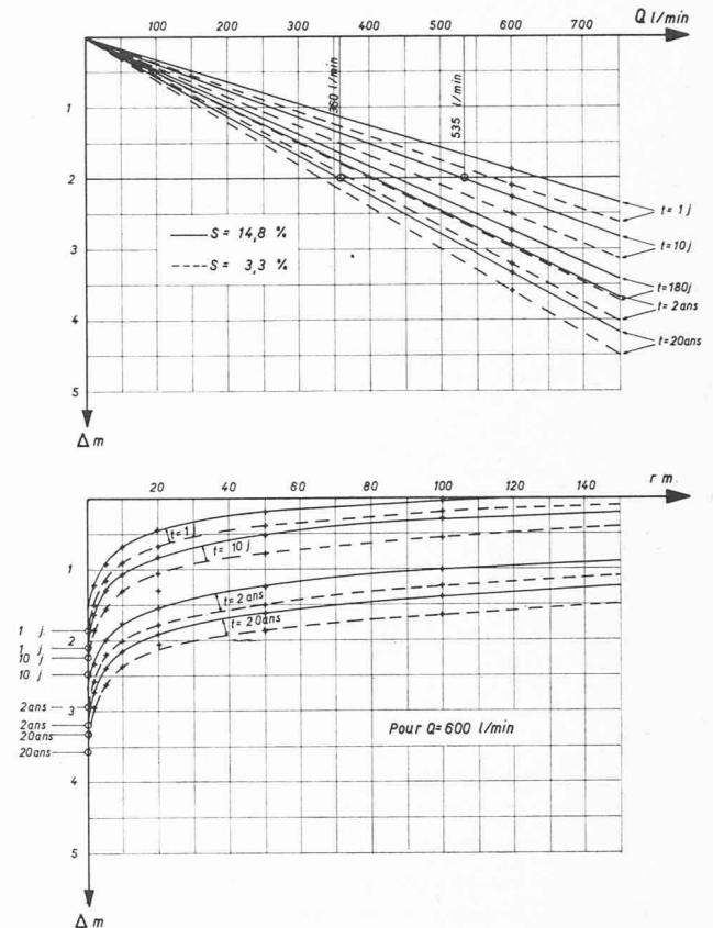
Fig. 18. — Puits d'essai de Cressier : droites caractéristiques \Delta = f(Q) et courbes de dépression \Delta = f(r) .
