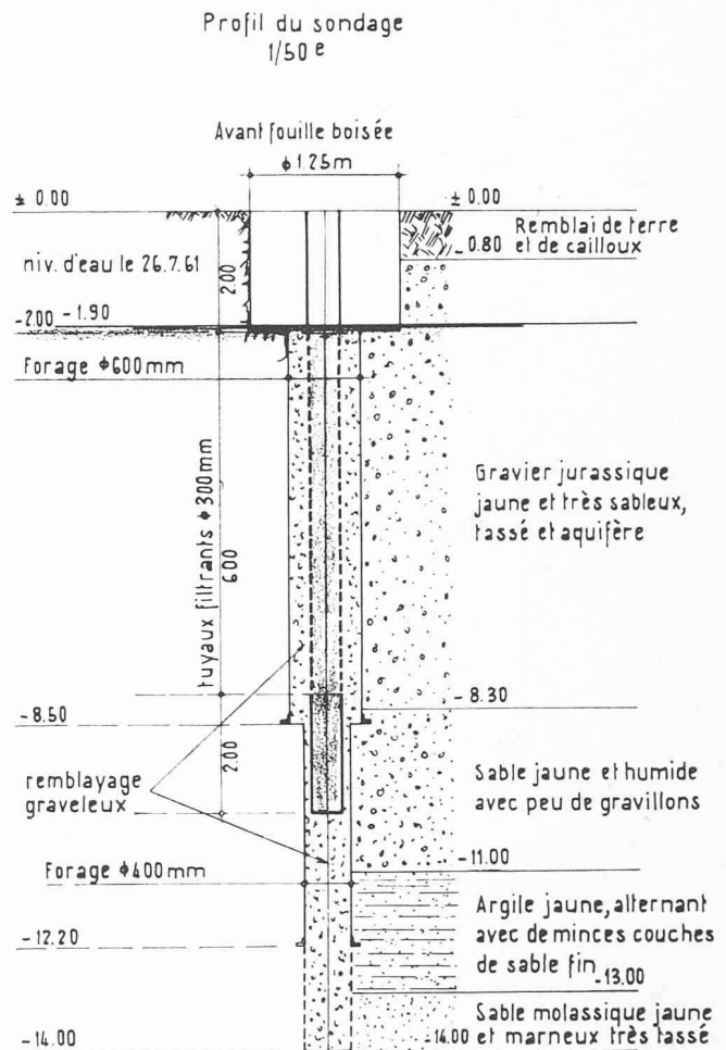
Fig. 14. — Coupe du puits d'essai.
