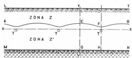
Fig. 13. — Drainage d'un terrain. Schéma du domaine.
