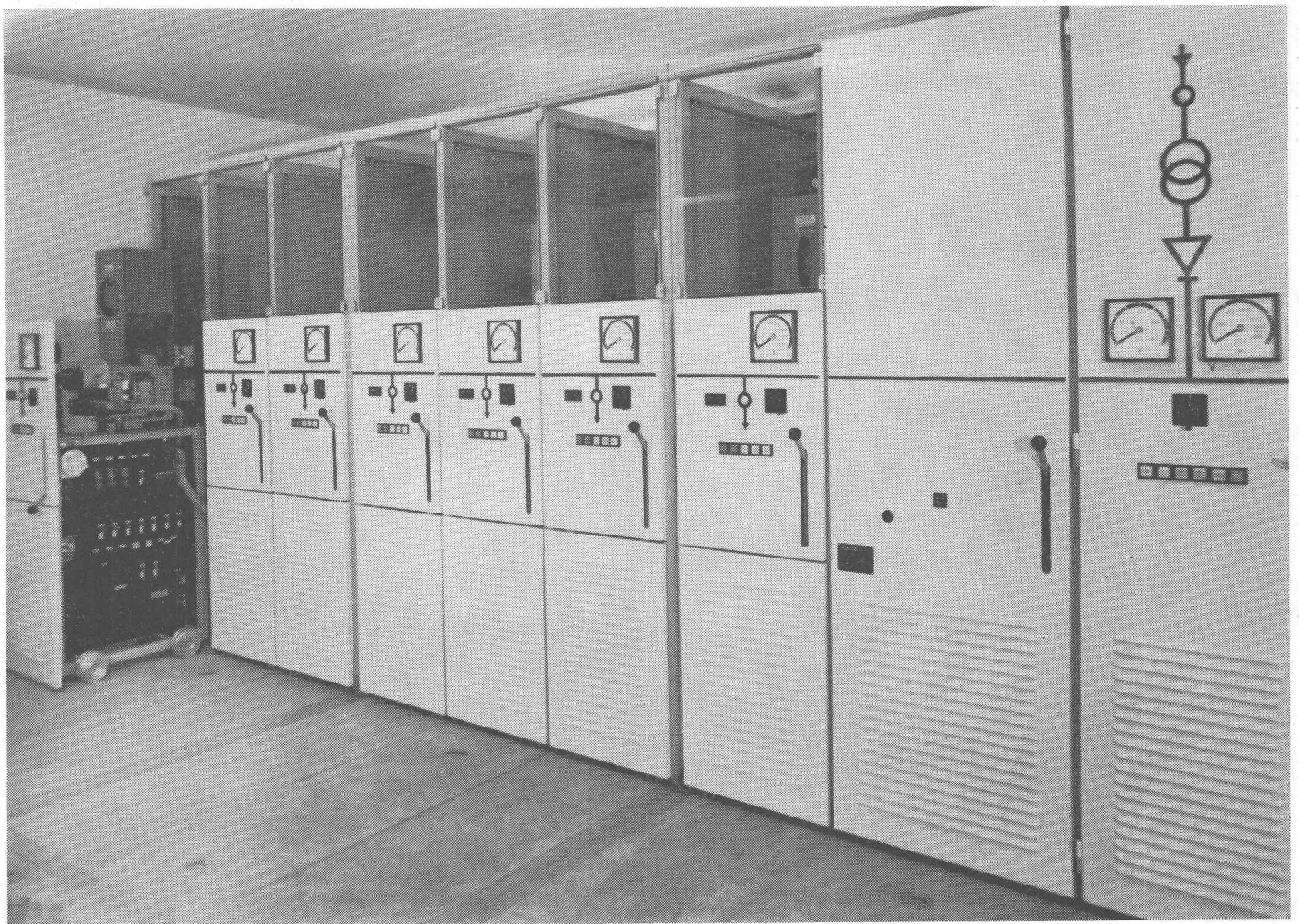
Sous-station de la Rudolfstrasse pour l'alimentation des tramways de la ville de Bâle.
