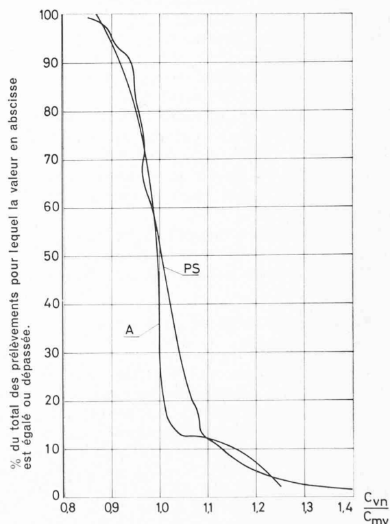
Fig. 4. — Variation des rapports \frac{C_{vn}}{C_{mv}} Porte-du-Scex et Carouge.
