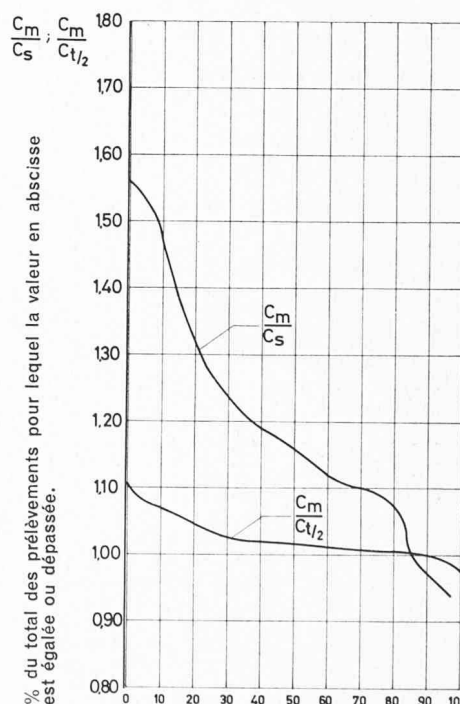
Fig. 1. — Variation des rapports \frac{C_m}{C_s} et \frac{C_m}{C_{t/2}} Porte-du-Scex - Rhône. 88 observations.
