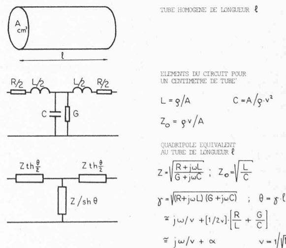
Fig. 12. — Tube de longueur arbitraire et l'un de ses circuits électriques équivalents.
