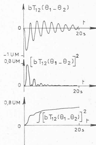
Fig. 6. — Paramètres : K_f = 4 ; K_t = 0,3 ; R = 0,16 . Influence du gain K_f — d^0
