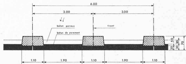
Fig. 3. — Mur ancré, coupe horizontale.
