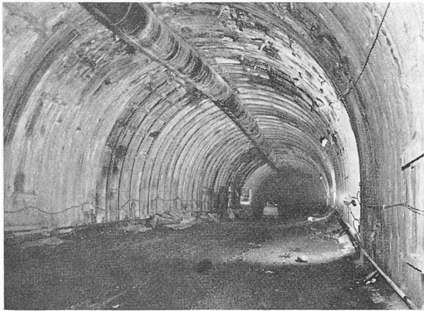
Fig. 10. — L'étayage métallique en cours de dépose.
