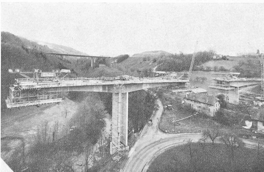
Fig. 8. — Vue en direction de la palée 2 et de la culée côté Montreux.
