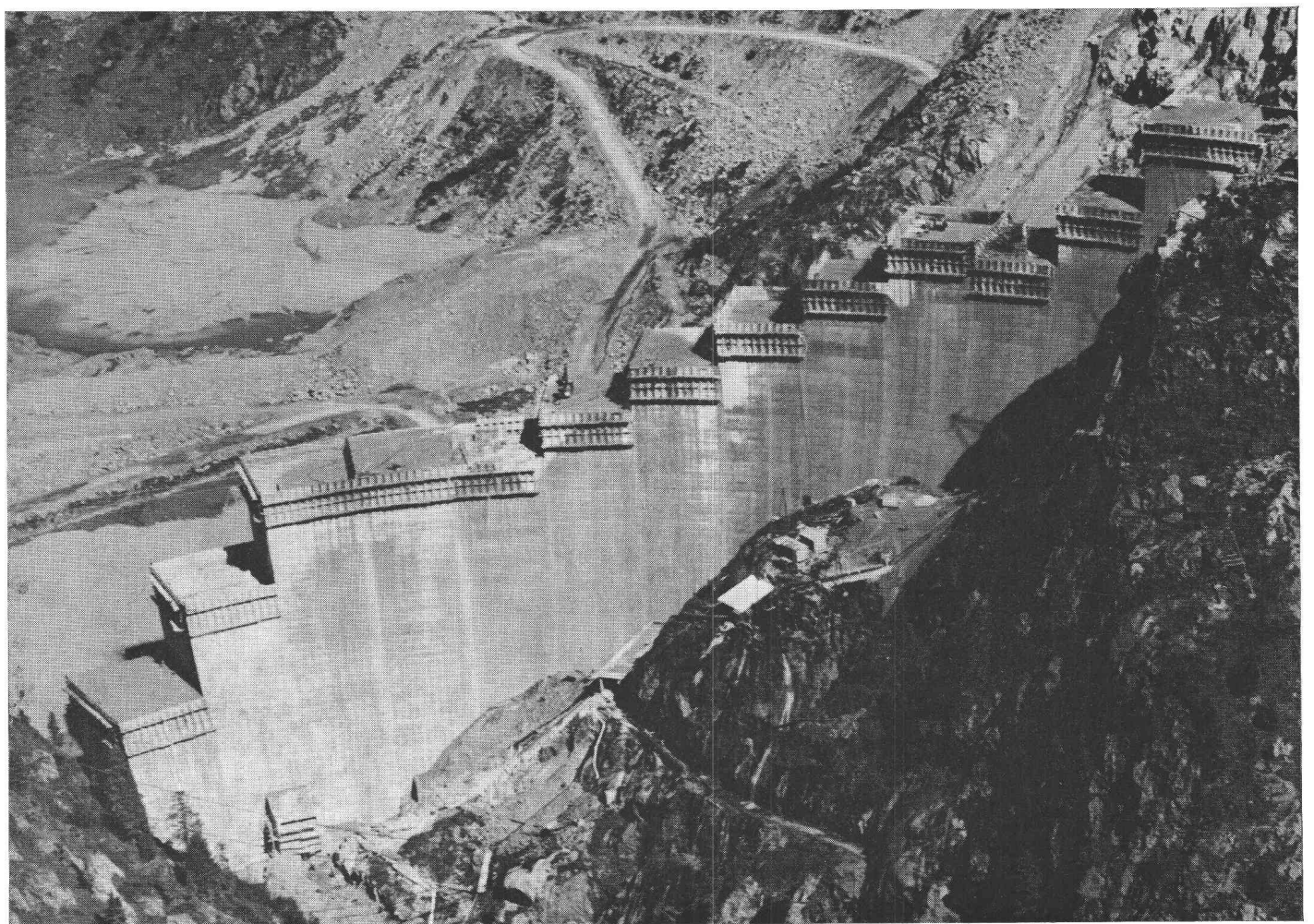
Barrage d'Emosson d'Electricité d'Emosson S. A. à Martigny. Etat des travaux en août 1971.
