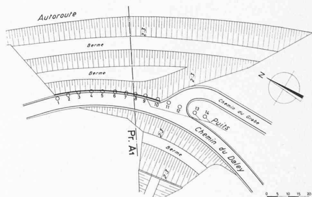
Fig. 8. — Plan de situation des puits.
