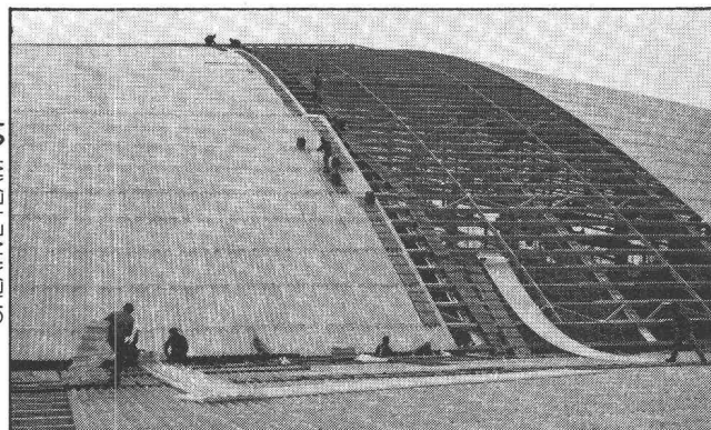
Toit vitré de neomat, patinoire de Berne
