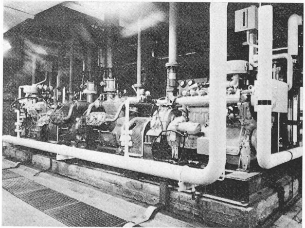
Fig. 2. — Le cœur de la pompe thermodynamique : à droite un des deux moteurs à gaz, à gauche un des deux compresseurs pour la réfrigération.
