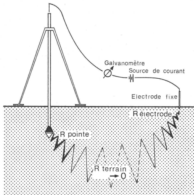
Schéma de principe du pénétromètre-électrode
