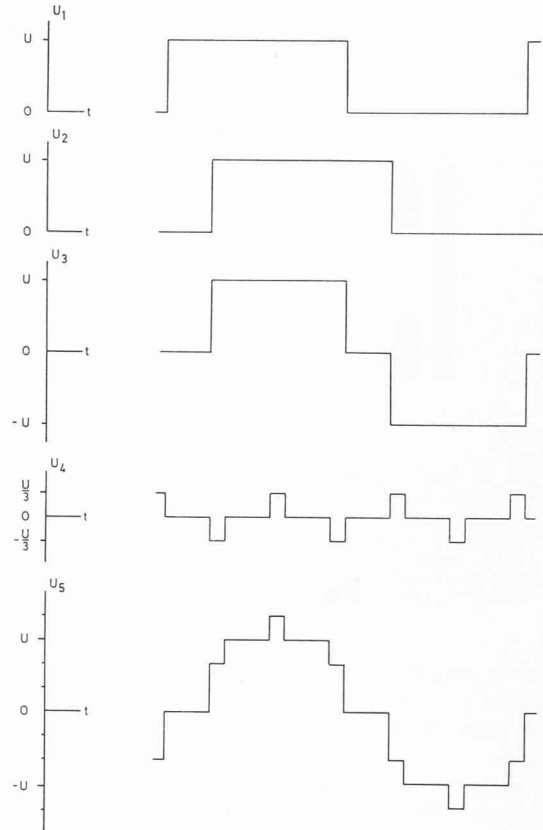
Fig. 205. — Séquences des tensions d'une phase d'un onduleur triphasé à double pulsation dans le procédé de la commande rectangulaire.
