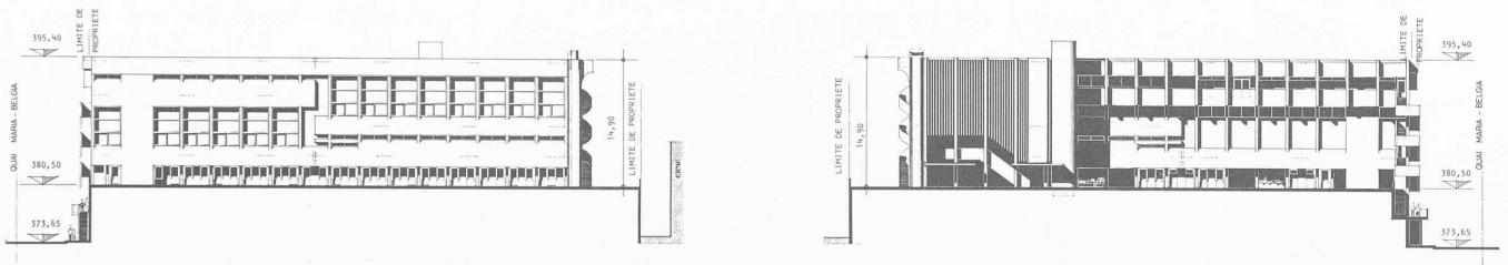
Fig. 9. — Bâtiment communal. Façade est (à gauche) et ouest (à droite).
