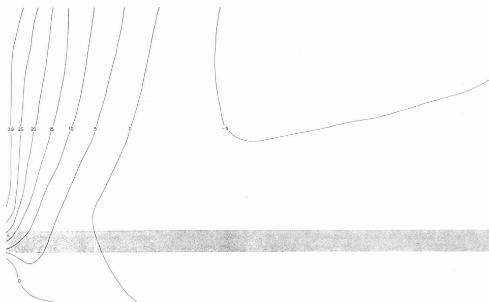
Fig. 3. — Cas n° 1 : \tau_{xy} .
