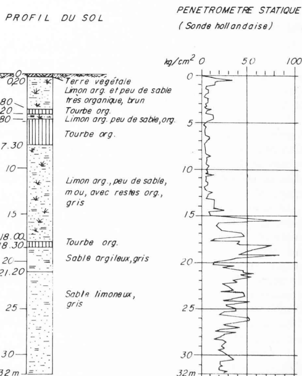
Fig. 2. — Profil du sol et diagramme de pénétration statique.
