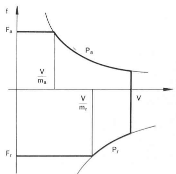
Fig. 2. — Poussée spécifique en fonction de la vitesse d'un propulseur à puissance constante.
