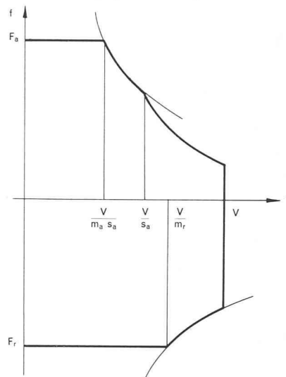
Fig. 1. — Poussée spécifique en fonction de la vitesse d'un propulseur de type série.
