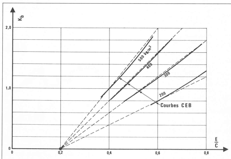
Fig. 8. — Paramètre K_b en fonction du rapport E/C pour différents dosages (d'après CEB-FIP).
