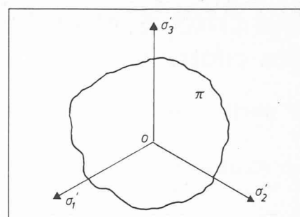
Fig. 3.5. — Projection des axes \sigma_1 , \sigma_2 et \sigma_3 sur le plan \pi .
