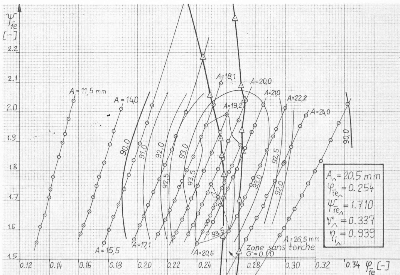
Fig. 3. — Colline de rendement du modèle réduit des turbines de LG 2.
